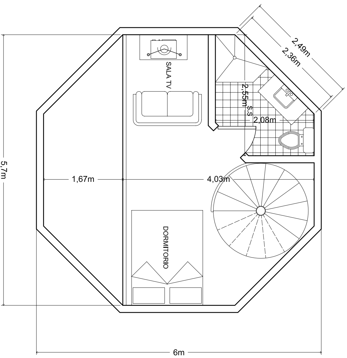
APARTAMENTO #2 PLANTA ALTA PROPUESTA - 1
