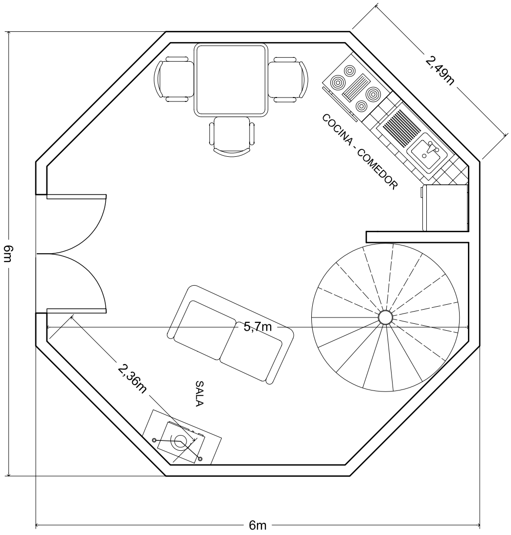
APARTAMENTO #2 PLANTA BAJA PROPUESTA - 1
